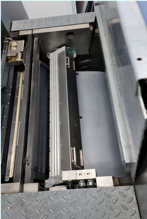
HEIDELBERG XL 75 INTERDECK UNIT
